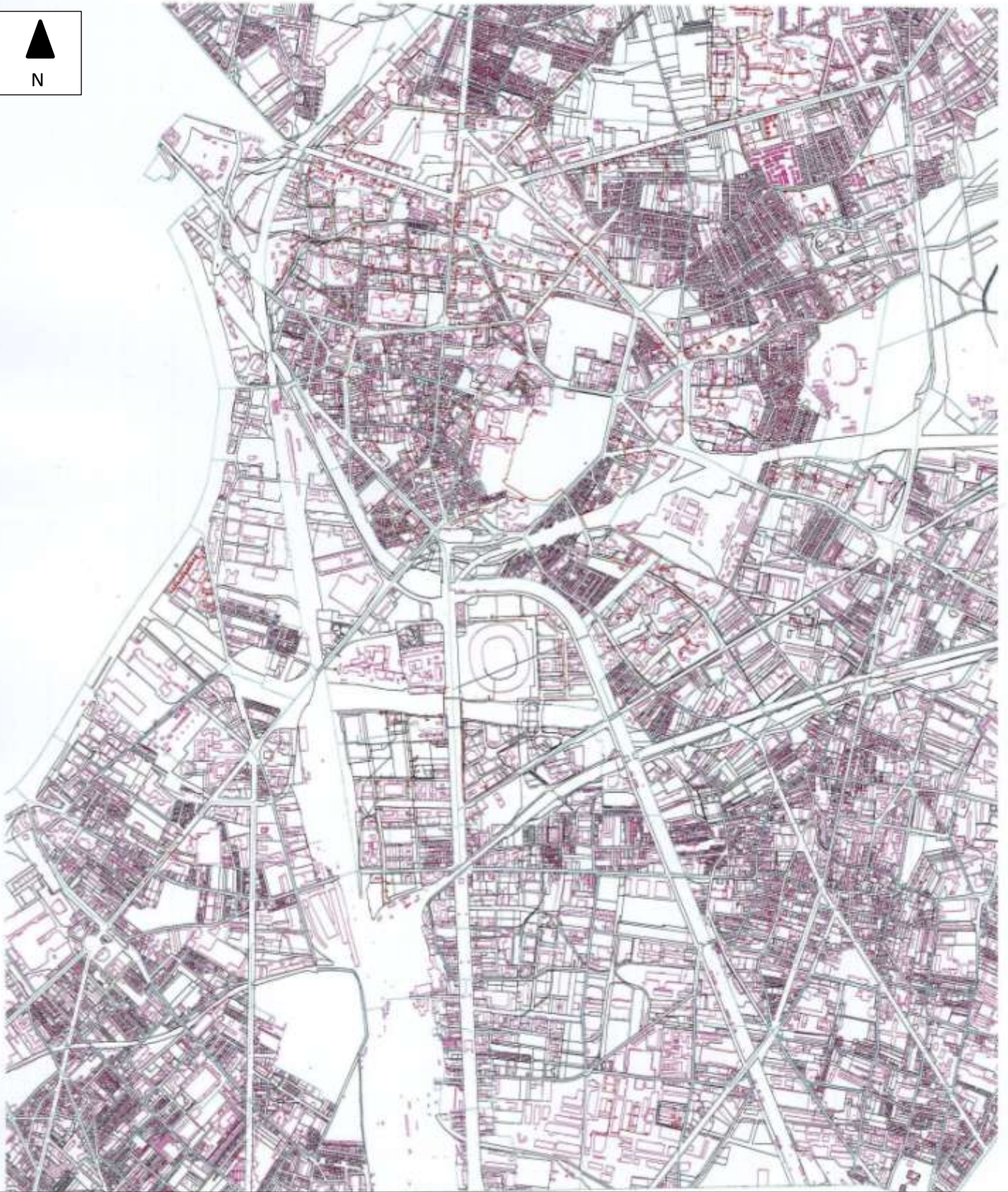
PLAN DE RESEAU DU CHAUFFAGE URBAIN –VILLE DE SAINT-DENIS
