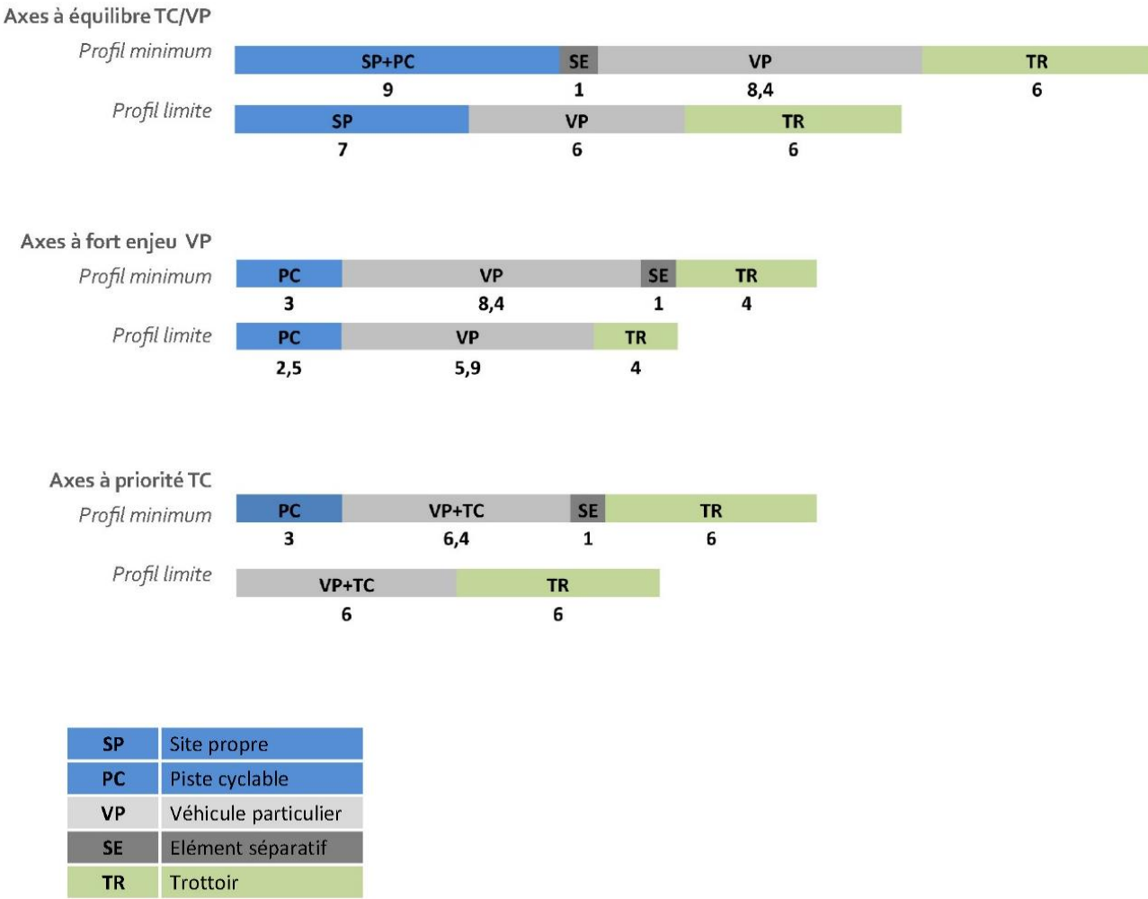
Figure n° 1 : Profils-types de voiries en fonction du type d'axe
