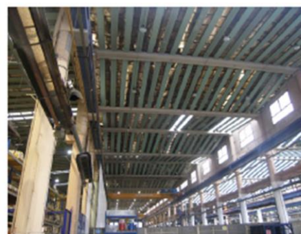
Halle en béton armé d'Alstom
